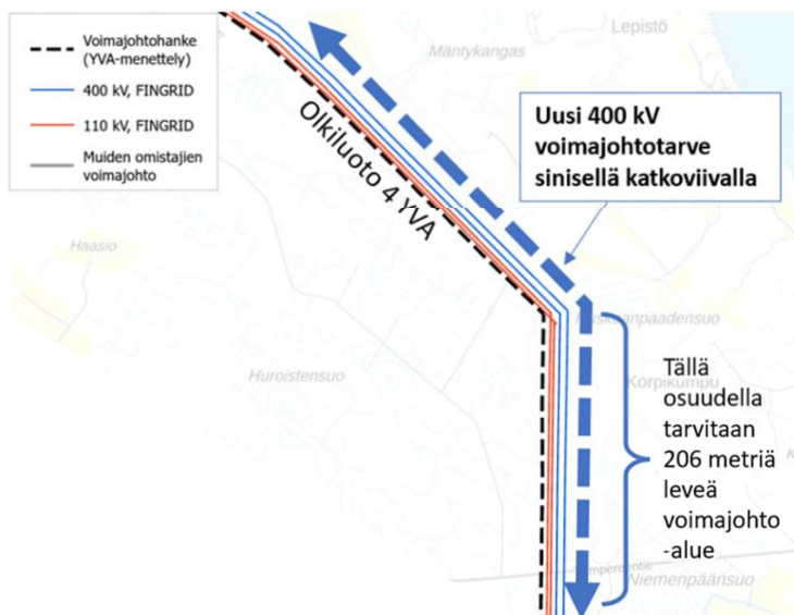
Kuva 7.11 Fingridin nykyiset voimajohtot ja voimajohtojen kehittämistarpeet.
